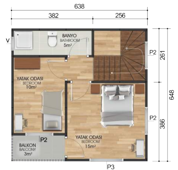
1. Kat Planı / First Floor PLAN 38m 2 + 3m 2 = 41m 2
